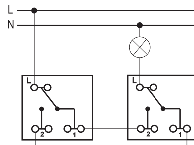
Schemat podłączenia dwóch łączników schodowych.
