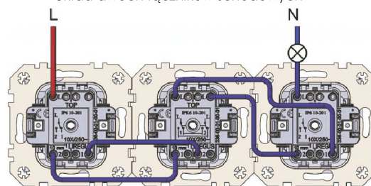
Układ dwóch łączników schodowych z łącznikiem krzyżowym.
