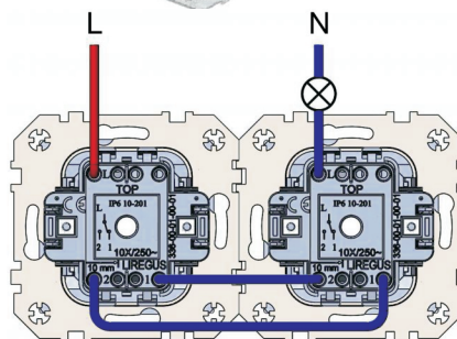
Układ dwóch łączników schodowych
